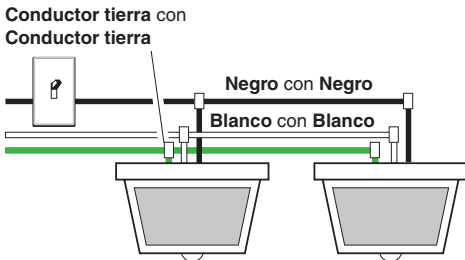
Dos lámparas detectoras de movimiento (trabajando de independientemente)
